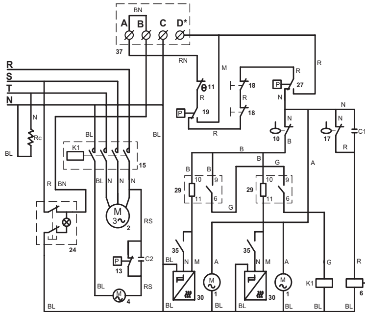
VERSIONE AD ARIA / AIR COOLED
