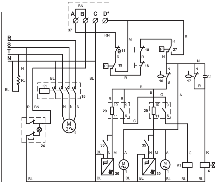
VERSIONE AD ACQUA / WATER COOLED
